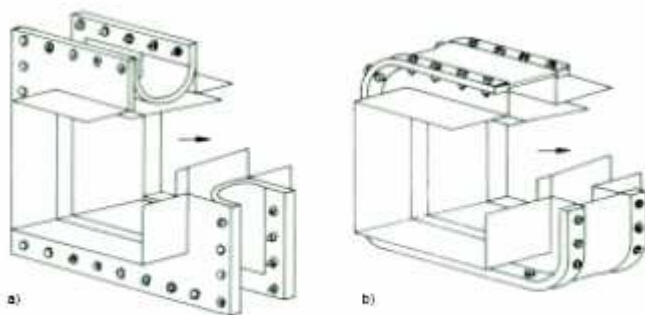
Bild 1 Bauarten von Weichstoffkompensatoren a) U-Kompensator b) Flanschbandkompensator
