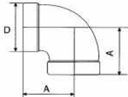
· Elbow 90° F/F Ref. 2001
